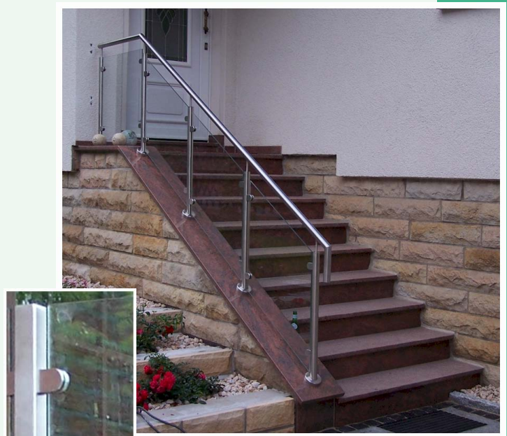
02 Edelstahlgeländer VSG-Füllung mit Einzelglashaltern
