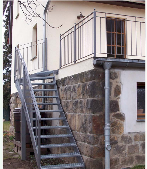
07 Flachstahlwangentreppe 1/4 gewendelt, Gitterroststufen, Stabgeländer, feuerverzinkt
