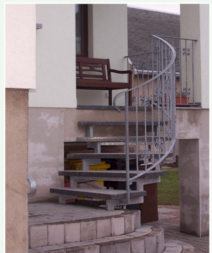
2-Holmtreppe 1/4 gewendelt, Natursteinstufen, schmiedeeisenes Geländer feuerverzinkt
